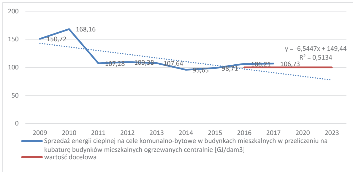
Rys. 7. Sprzedaż energii ciepłej na cele komunalno-bytowe w budynkach mieszkalnych w przeliczeniu na kubaturę budynków mieszkalnych ogrzewanych centralnie [GJ/dam³].
